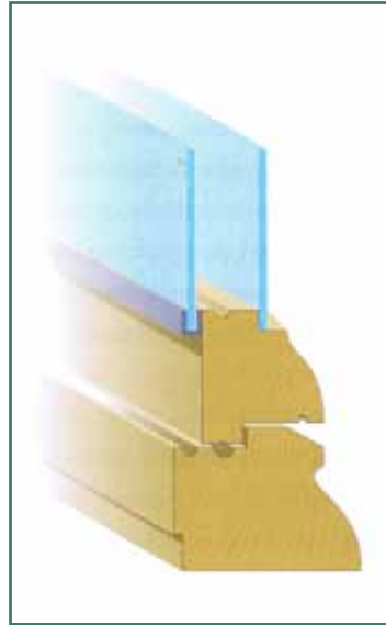
Voorzetbeglazing (bron: Bertrand J., Houten schrijnwerk; erfgoed en comfort verenigen, BROH-Directie Monumenten en landschappen, 2005, p. 37).
